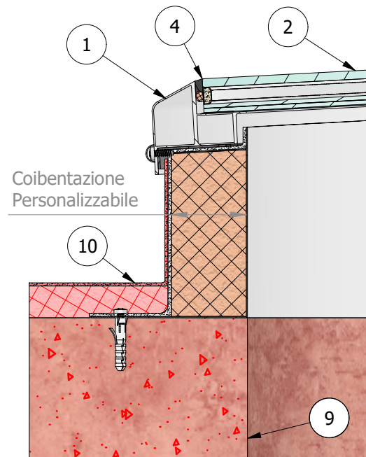
SU BASAMENTO SENZA GOCCIOLATOIO
