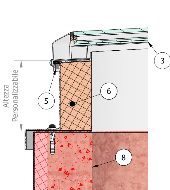
SU BASAMENTO CON GOCCIOLATOIO
