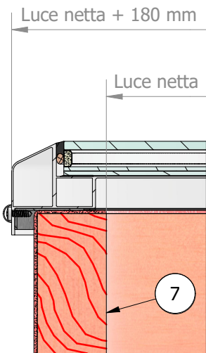
ANTA SU CORDOLO O BASAMENTO ESISTENTE
